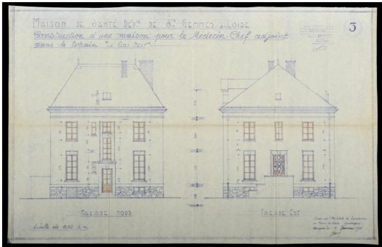
Construction d'une maison pour le Médecin-Chef-adjoint dans le terrain ""Le clos neuf"". Façade nord et façade est, par Ernest Bricard. 1928. (Archives départementales de Maine-et-Loire, 4 N).
