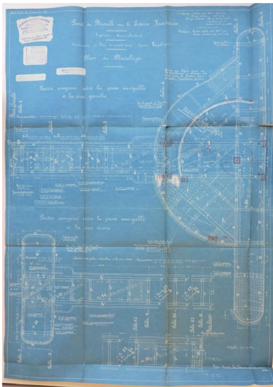
Dessin d'exécution des travaux de construction du pont, plans de détail, 1912.
