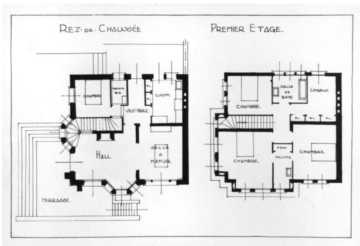
Plans de la villa La Rigaudière 2.
