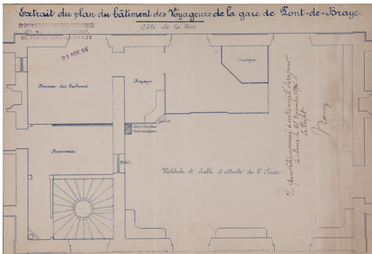
Extrait du plan du bâtiment des voyageurs de la gare de Pont-de-Braye, 1894.
