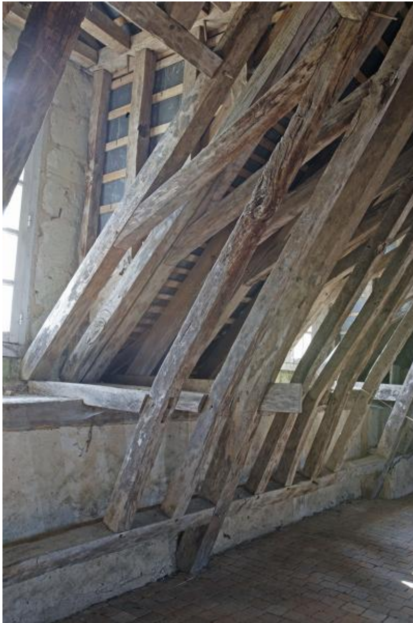
Le grand comble et sa charpente, chevrons, arbalétriers et blochets.
