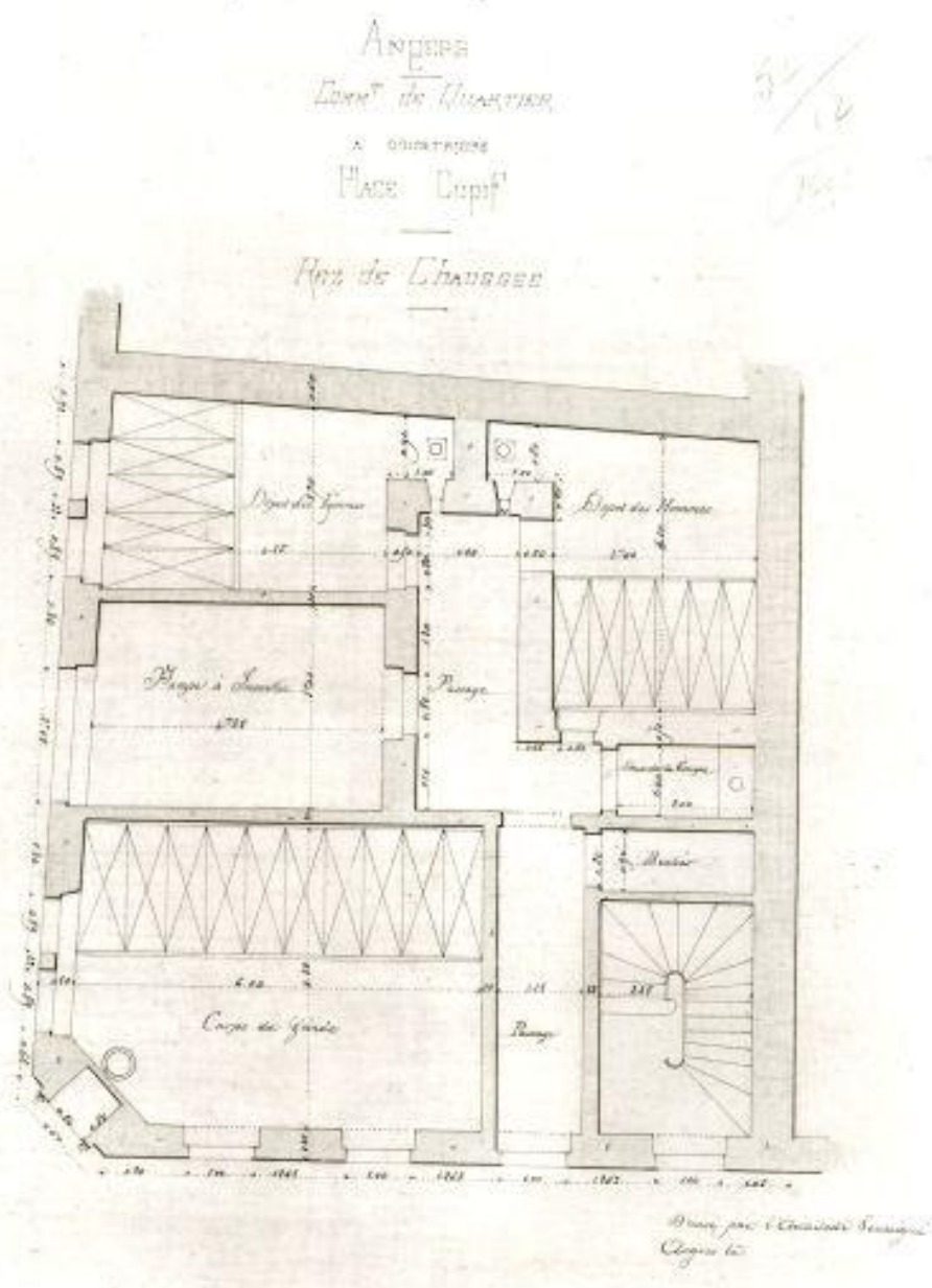
Angers. Commissariat de Quartier à construire Place Cupif. Rez- de- chaussée, dessin, par E. Dainville, [1870]. (Archives départementales de Maine-et-Loire ; 90 J 491).
