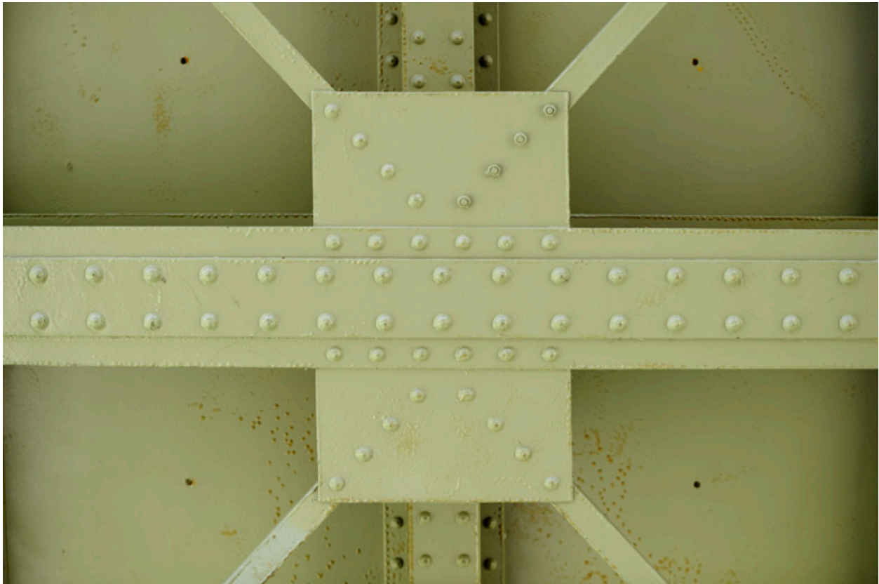
Charpente métallique soutenant le tablier (détail)
