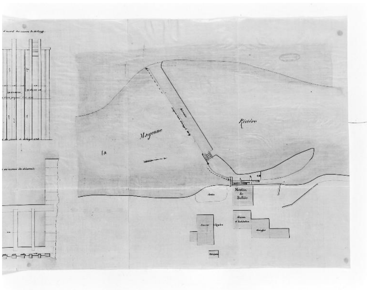
Plan-masse du moulin, de ses dépendances et du barrage, 1863.
