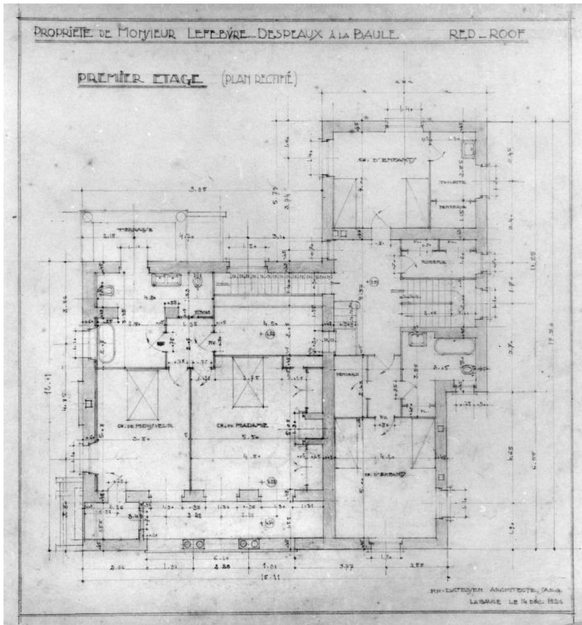
Plan du 1er étage au 1/50e de la villa Red-Roof pour M. Lefebvre Despeaux en 1926.
