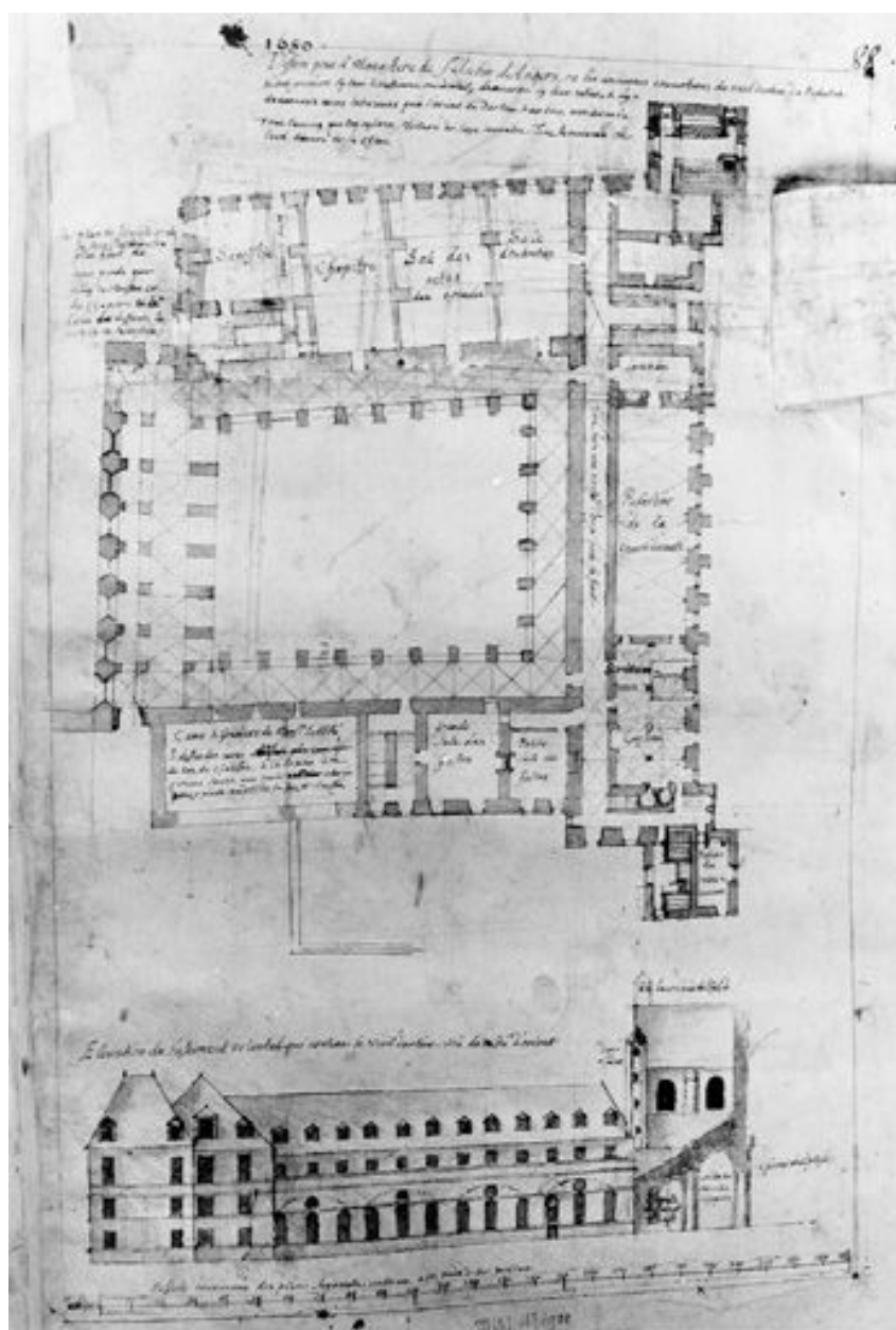
Projet global de reconstruction, attribué à Marc Rivard : plan du rez-de-chaussée (version sans le rabat) et élévation sur jardin de l'aile orientale des dortoirs, 1680. (Bibliothèque municipale de Meaux ; Ms. 44, f. 88 v°).
