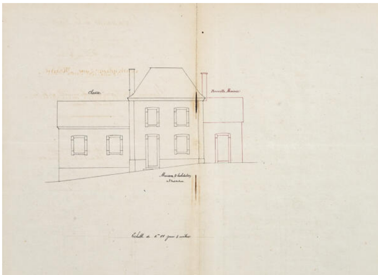
Mairie-école de Montreuil-le-Henri : plan en élévation, 1874.
