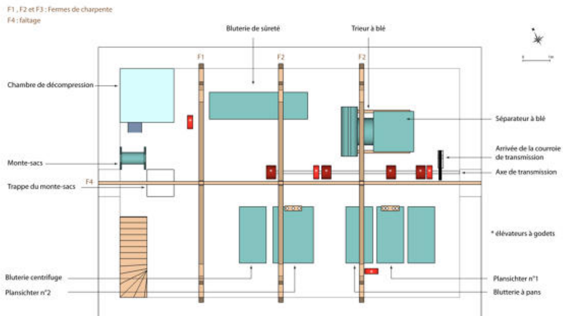
SAINT-SULPICE (53) - Moulin de la Rongère Plan schématique du comble, en partie restitué.
