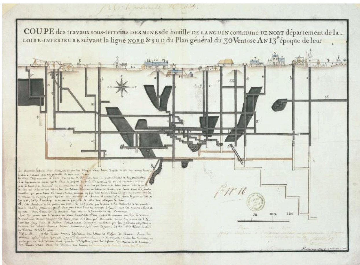
Coupe des travaux souterrains, an 13.
