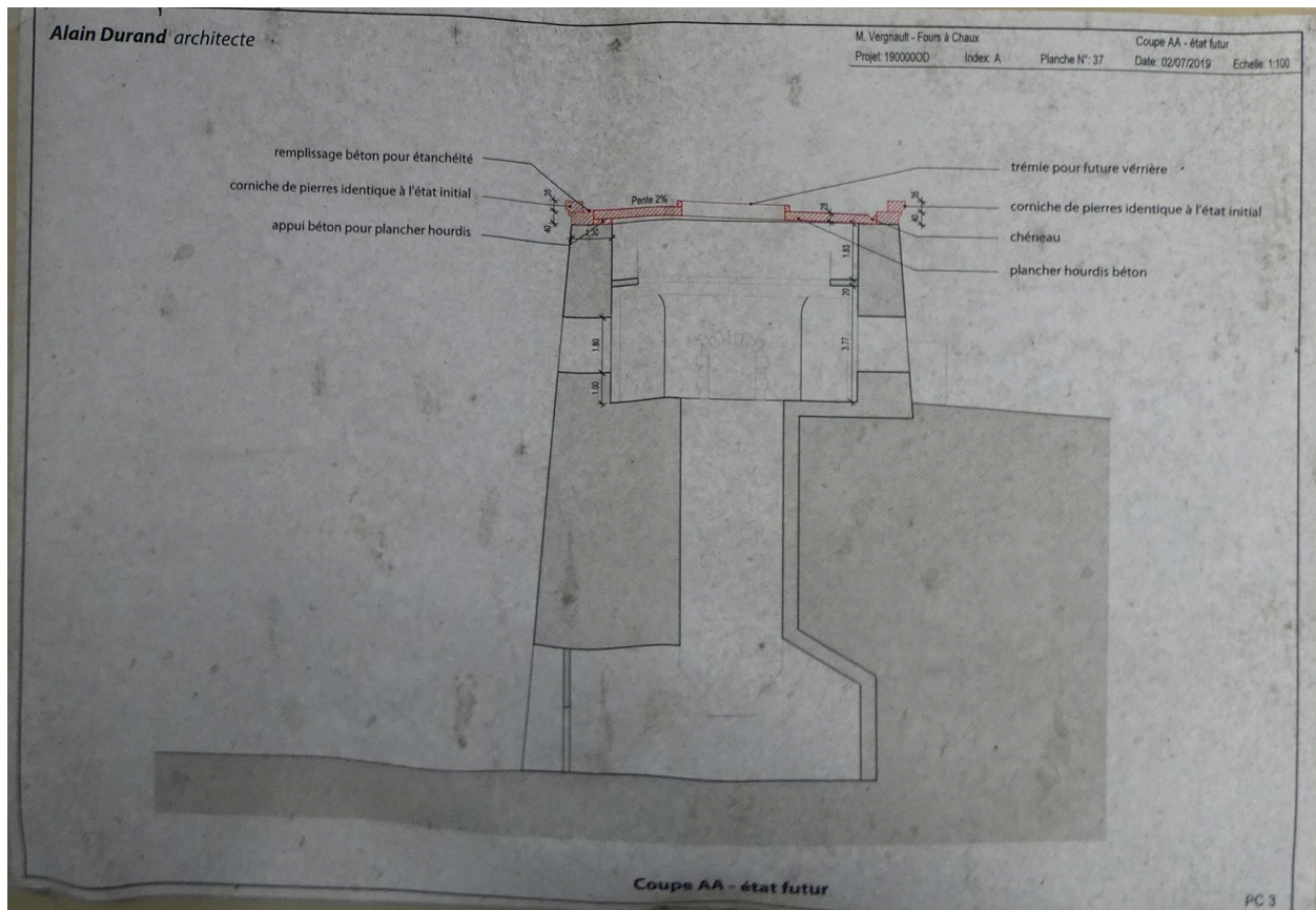
Coupe d'un des fours, par l'architecte Alain Durand, en 2019.
