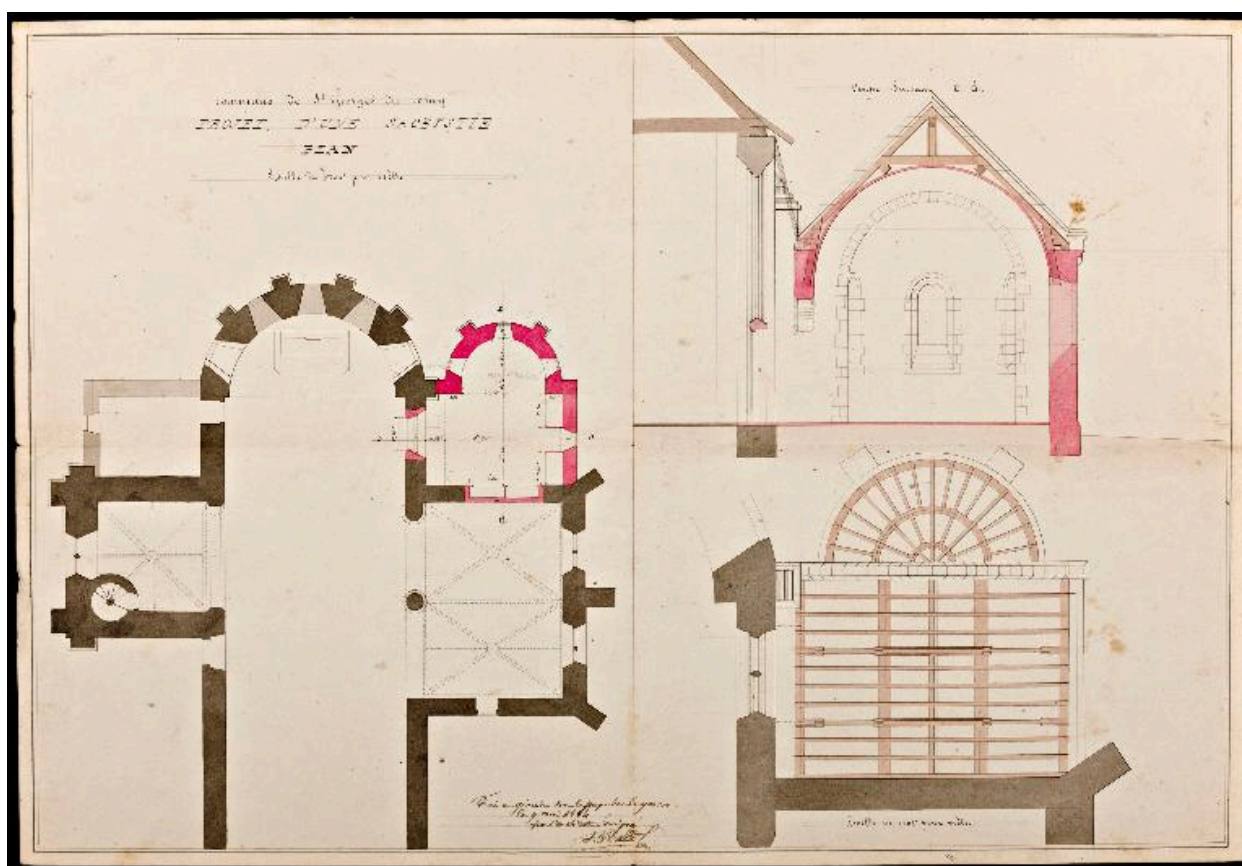
Plans et coupe du projet de sacristie néo-romane non réalisé. 1864.
