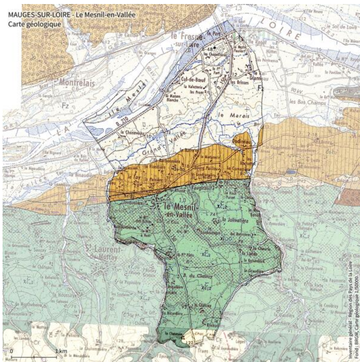
Le Mesnil-en-Vallée. Carte géologique au 1/50 000e. (c) BRGM.
