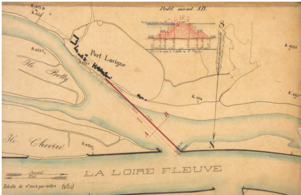
Plan joint au projet de digue à construire sur la rive gauche du bras de Port-Lavigne, 1892.
