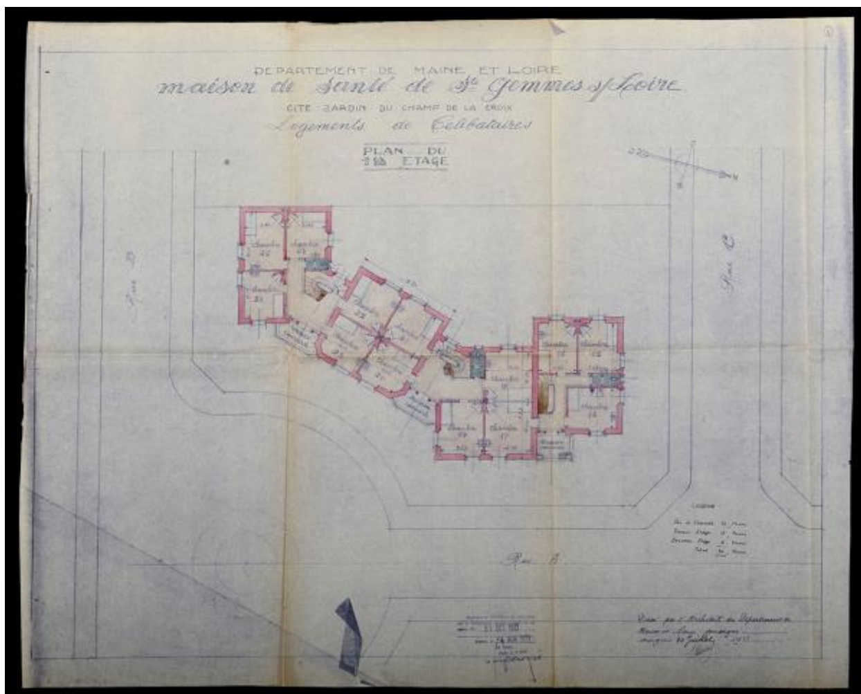
Logements pour célibataires. Plan d'un étage, par Ernest Bricard. Juillet 1934. (Archives départementales de Maine-et-Loire, 4 N).
