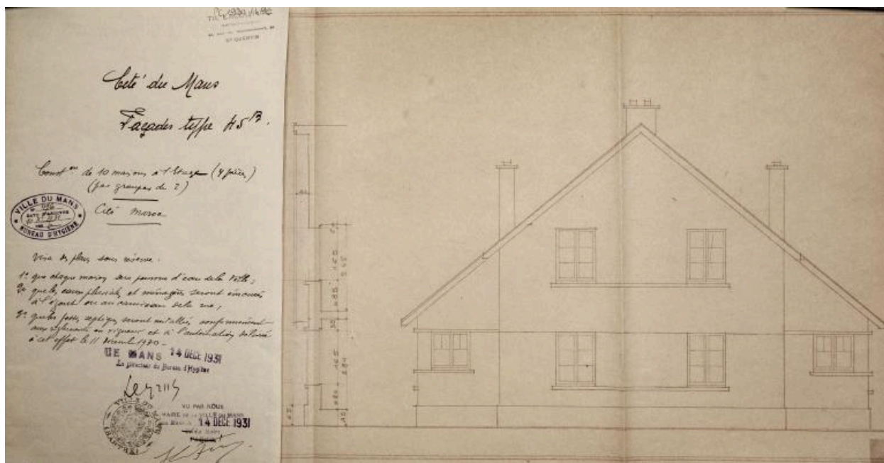
Elévation de la façade principale d'un pavillon de type 2, 1931.
