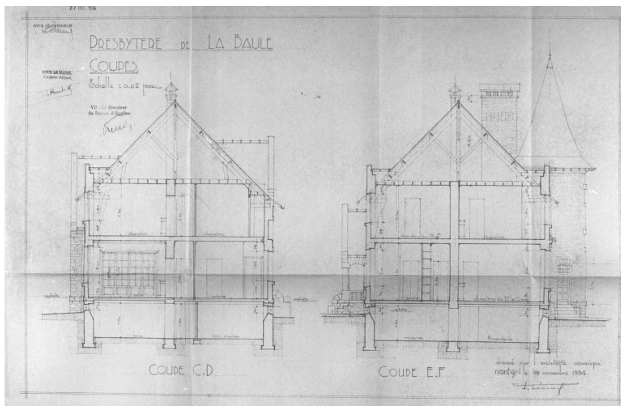
Presbytère de La Baule : coupes au 1/50e.
