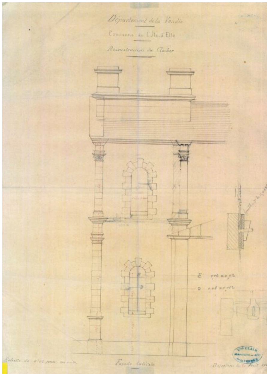
Projet de clocher par Victor Clair, 30 avril 1869 : élévation latérale sud.
