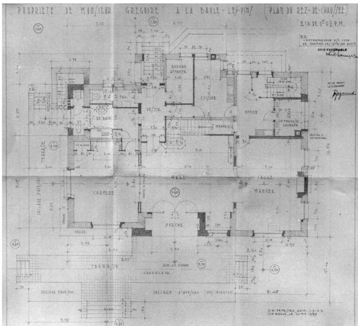
Plan du rez-de-chaussée au 1/50e de la villa Aktina.
