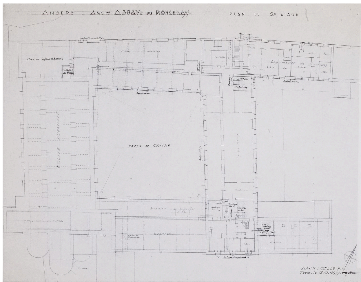
Ancienne abbaye du Ronceray. Plan du 2e étage, par René Baldet (recenseur MH). Tirage de plan, 1977, éch. 1 : 200. 41,5 x 54 cm.
