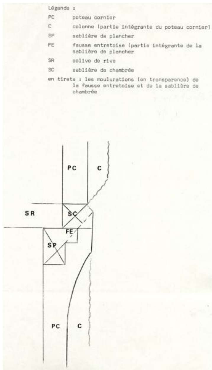
Coupe schématique d'un encorbellement.
