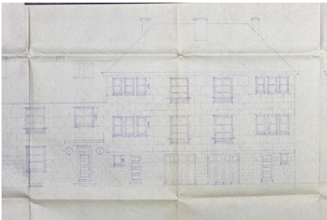
Elévation des façades des maisons du lotissement de la Prairie (détail).
