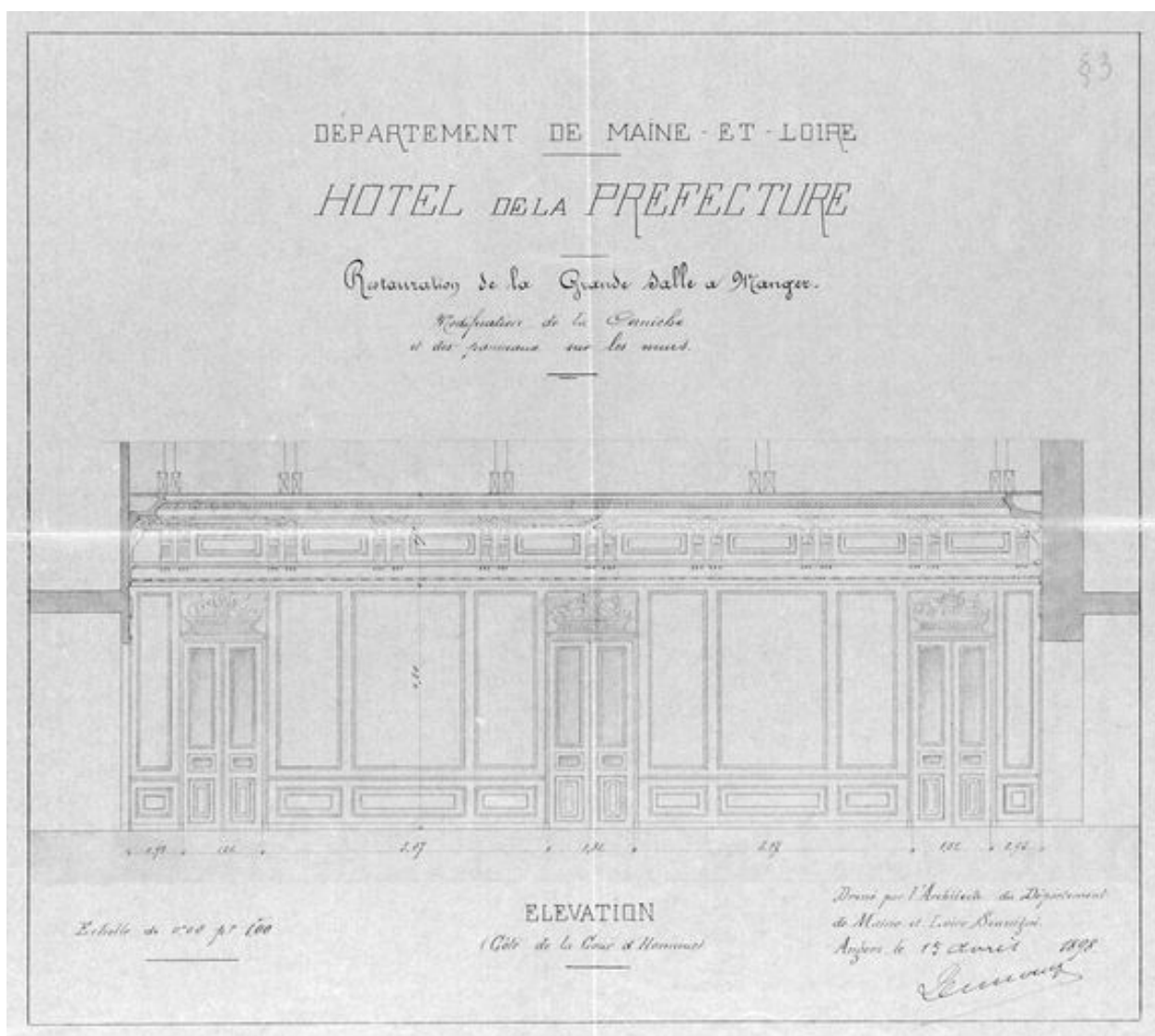
Département de Maine-et-Loire. Hôtel de la Préfecture. Restauration de la grande salle à manger. Modification de la corniche et des panneaux sur les murs. Elévation, par l'architecte Jules Dussauze, 1898. (Archives départementales de Maine-et-Loire ; N 1770).
