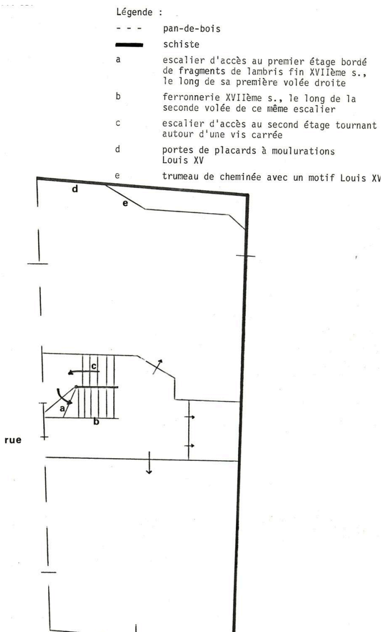
Plan schématique du premier étage.
