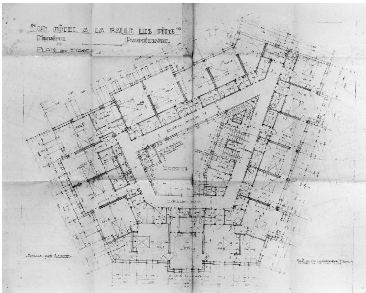
Plan des étages au 1/50e sur l'avenue Lajarrige (ancienne avenue des Tilleuls) de l'Hôtel des Palmiers
