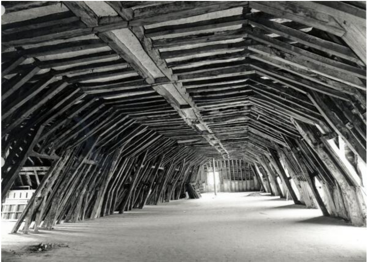
Aile ouest du cloître, étage de comble : vue d'ensemble de la charpente, de nord en sud.
