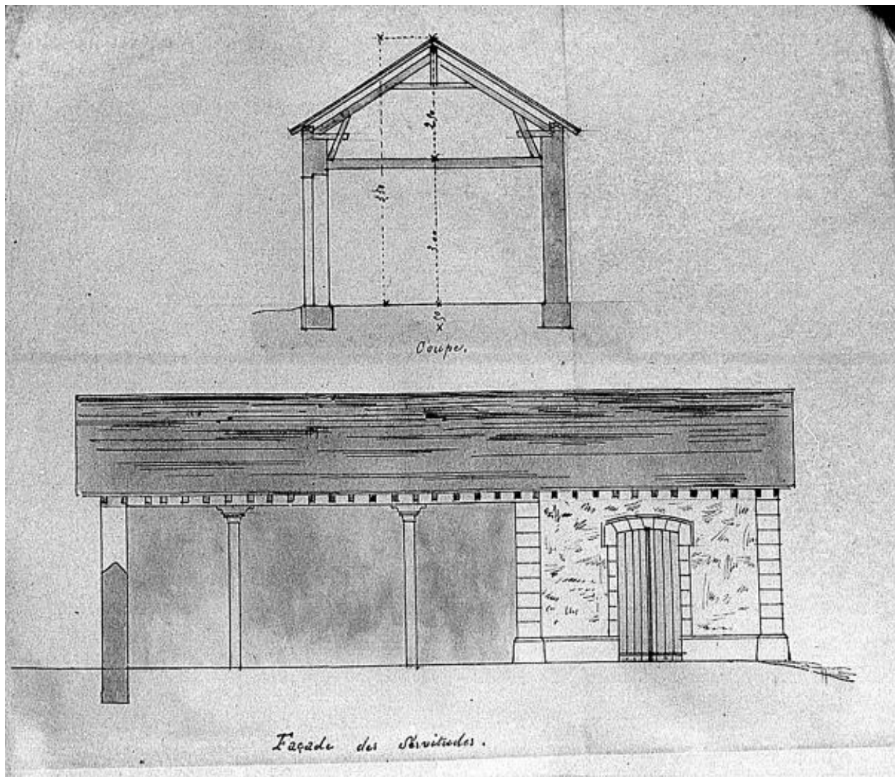
Plan des dépendances, Auguste Beignet, 1er avril 1876, échelle 1/100. (AM Montjean-sur-Loire ; 2 M 3).
