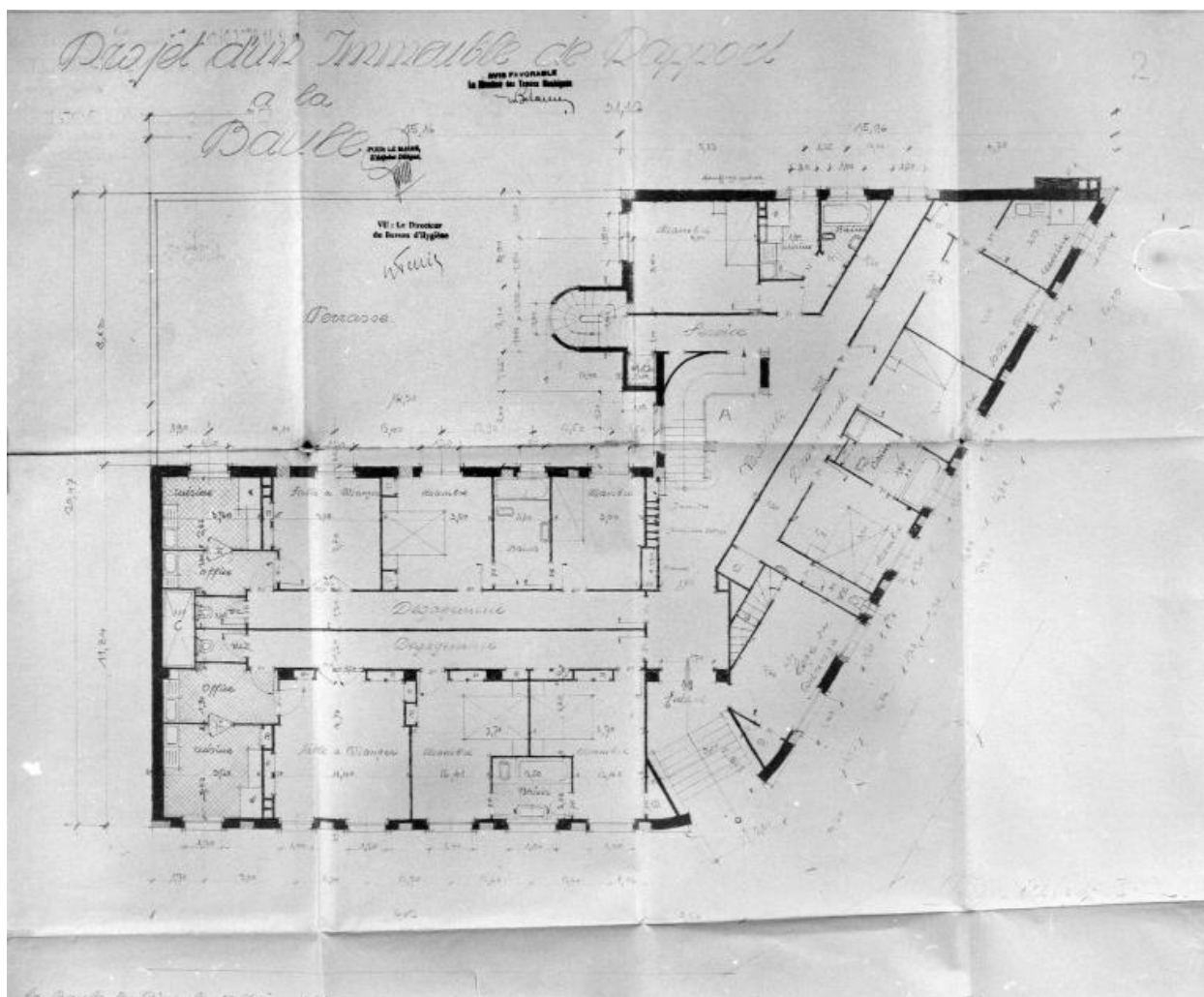
Plan du rez-de-chaussée au 1/50e du Bellevue Building.
