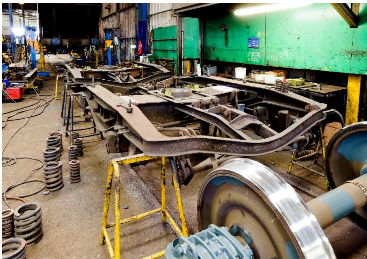
Atelier de réparation des bogies.
