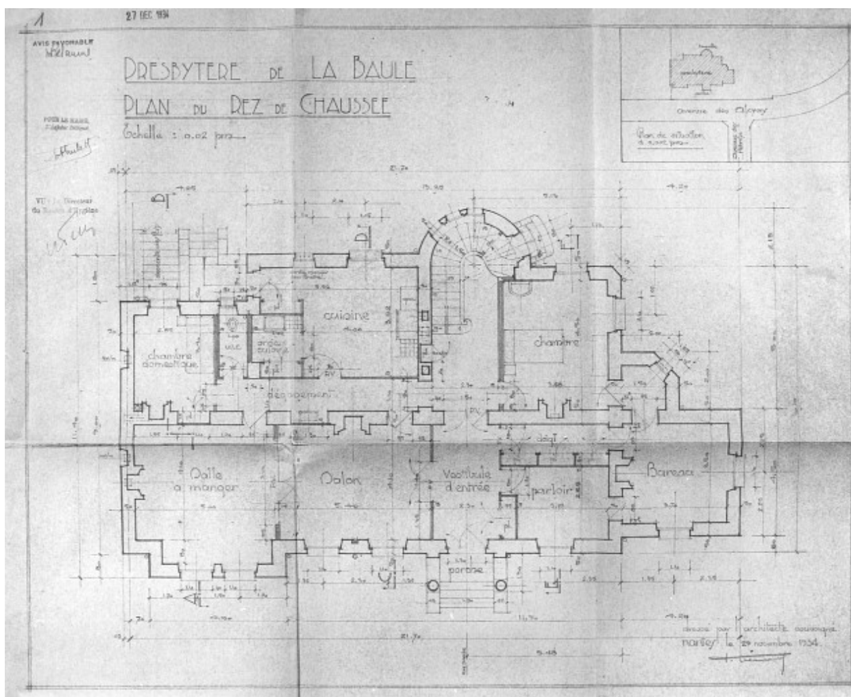
Presbytère de La Baule : plan du rez-de-chaussée au 1/50e.
