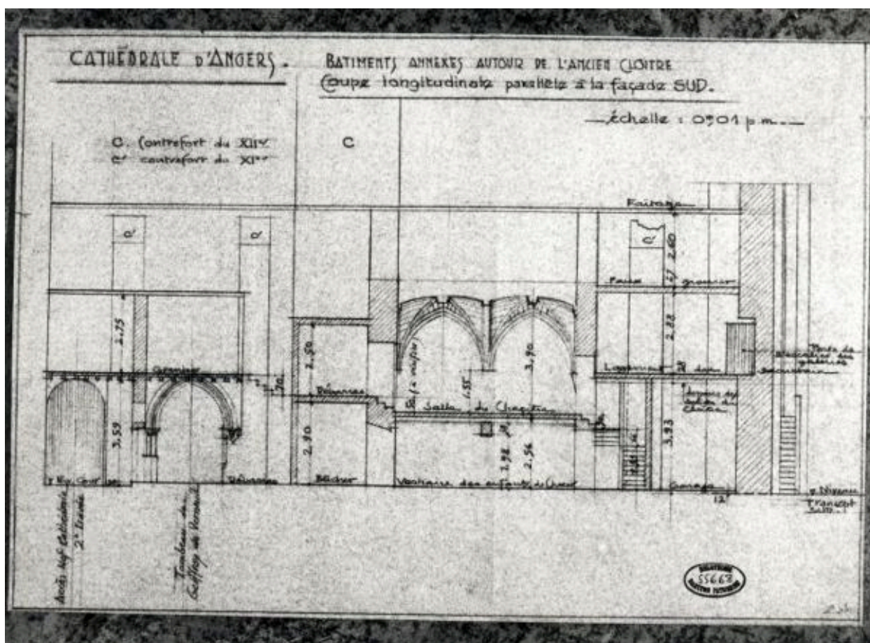
Bâtiments annexes autour de l'ancien cloître : coupe longitudinale parallèle au mur sud de la nef. Dessin, [v. 1950], éch. 1 : 100. 21 x 30,5 cm. (Médiathèque de l'Architecture et du Patrimoine ; 55668).
