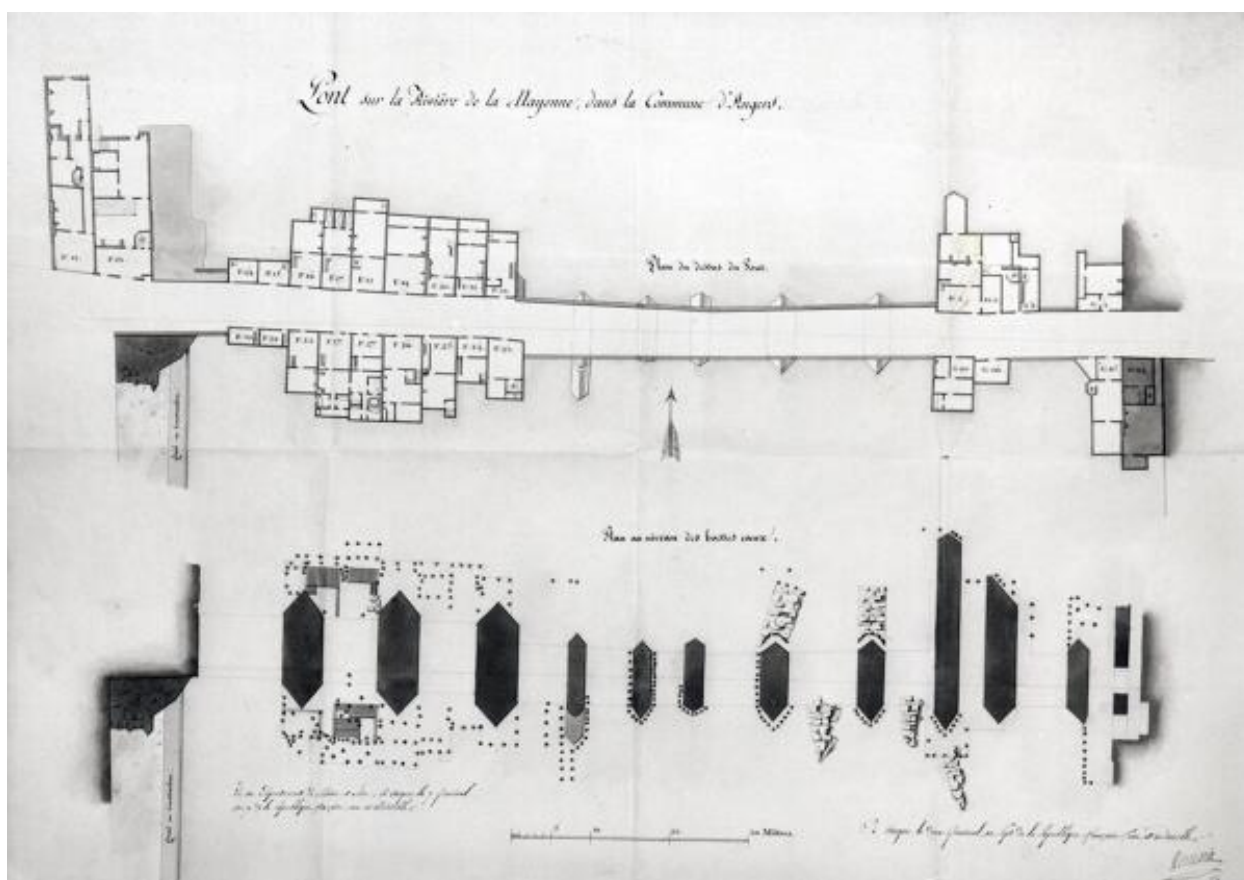
Pont sur la rivière de la Mayenne, dans la commune d'Angers. Plan du dessus du pont. Plan au niveau des basses eaux. Dessin à la plume et aquarelle, mars 1799, éch. 1 : 200 environ, par Jean-François Demarie (ingénieur ordinaire des Ponts et Chaussées), 1799. (Archives départementales de Maine-et-Loire ; 1 L 905).
