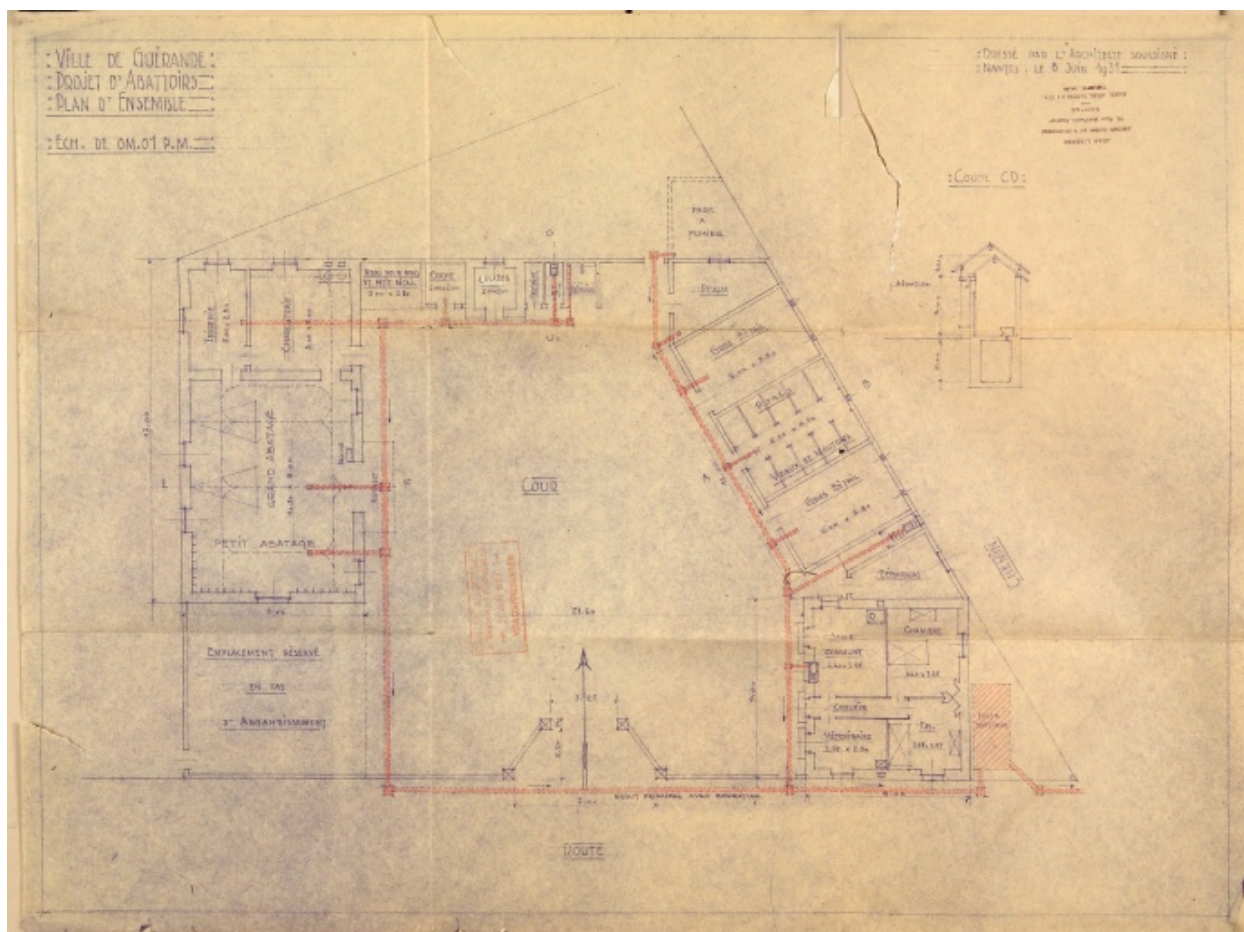
Plan de l'abattoir, projet de l'architecte Jean Liberge.
