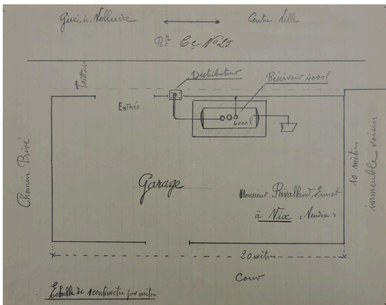
Plan d'installation du réservoir et de la pompe à essence, 1938.
