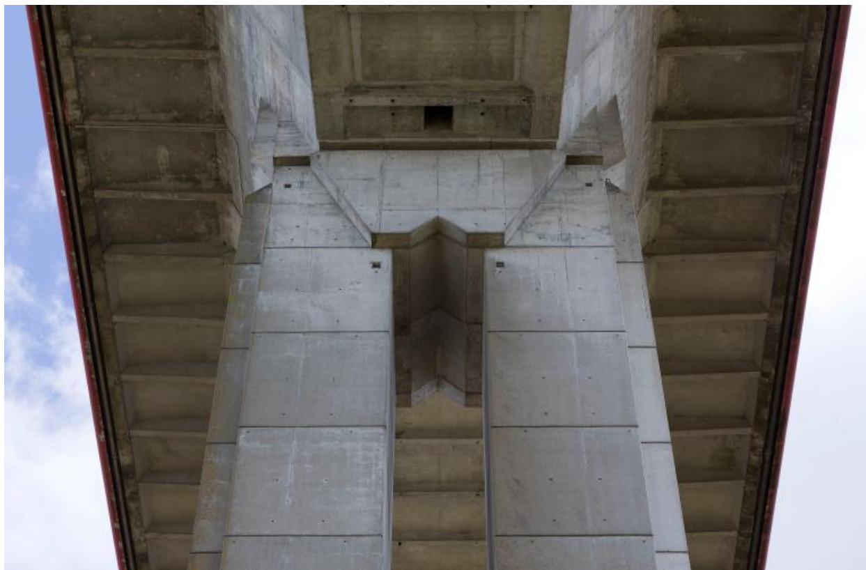
Détail d'une des deux piles principales soutenant le tablier central.
