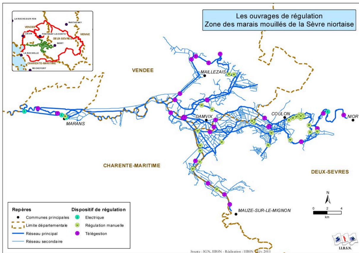
Carte des ouvrages de régulation des marais mouillés de la Sèvre Niortaise (source : IBSN).
