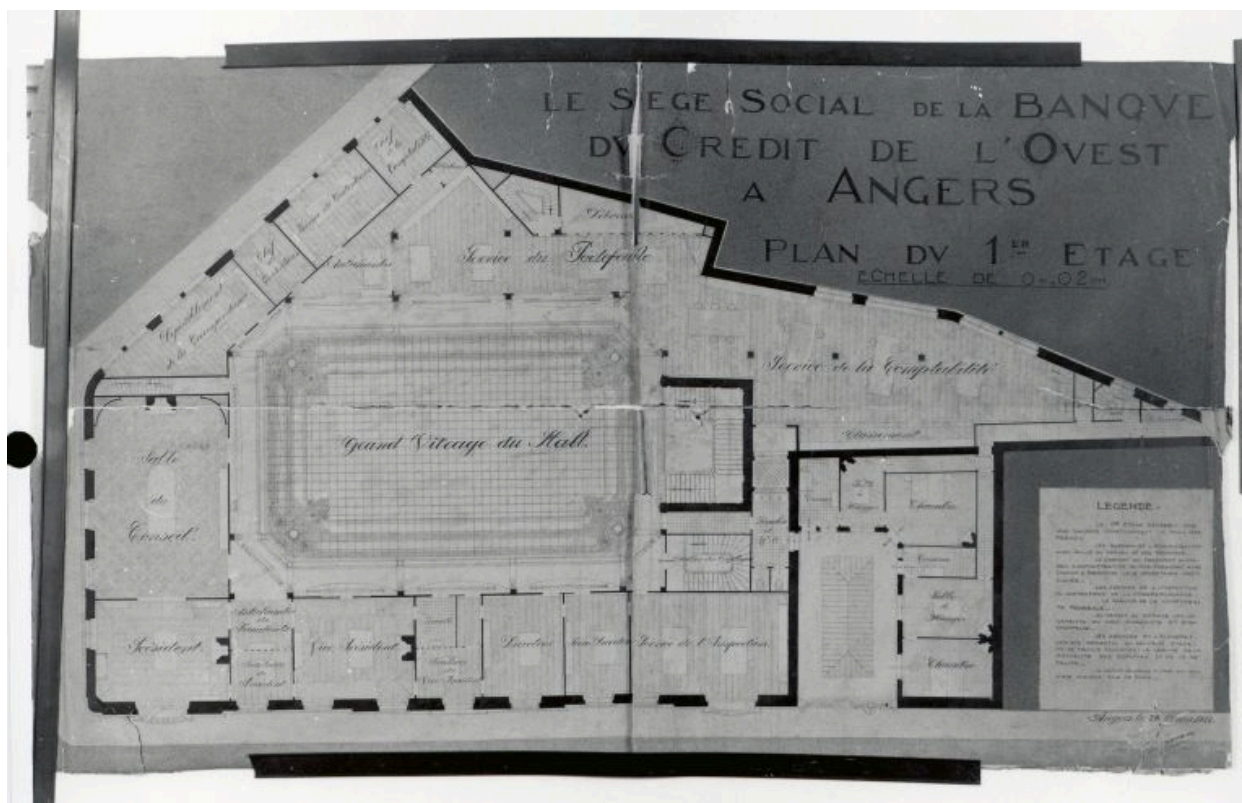
Le Siège Social de la Banque du Crédit de l'Ouest à Angers. Plan du 1er étage, par H. Jamard, [v. 1922].
