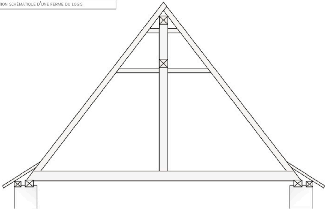
SAINT-JEAN-SUR-ERVE - Le Moulin-aux-Moines ÉLÉVATION SCHÉMATIQUE D'UNE FERME DU LOGIS
