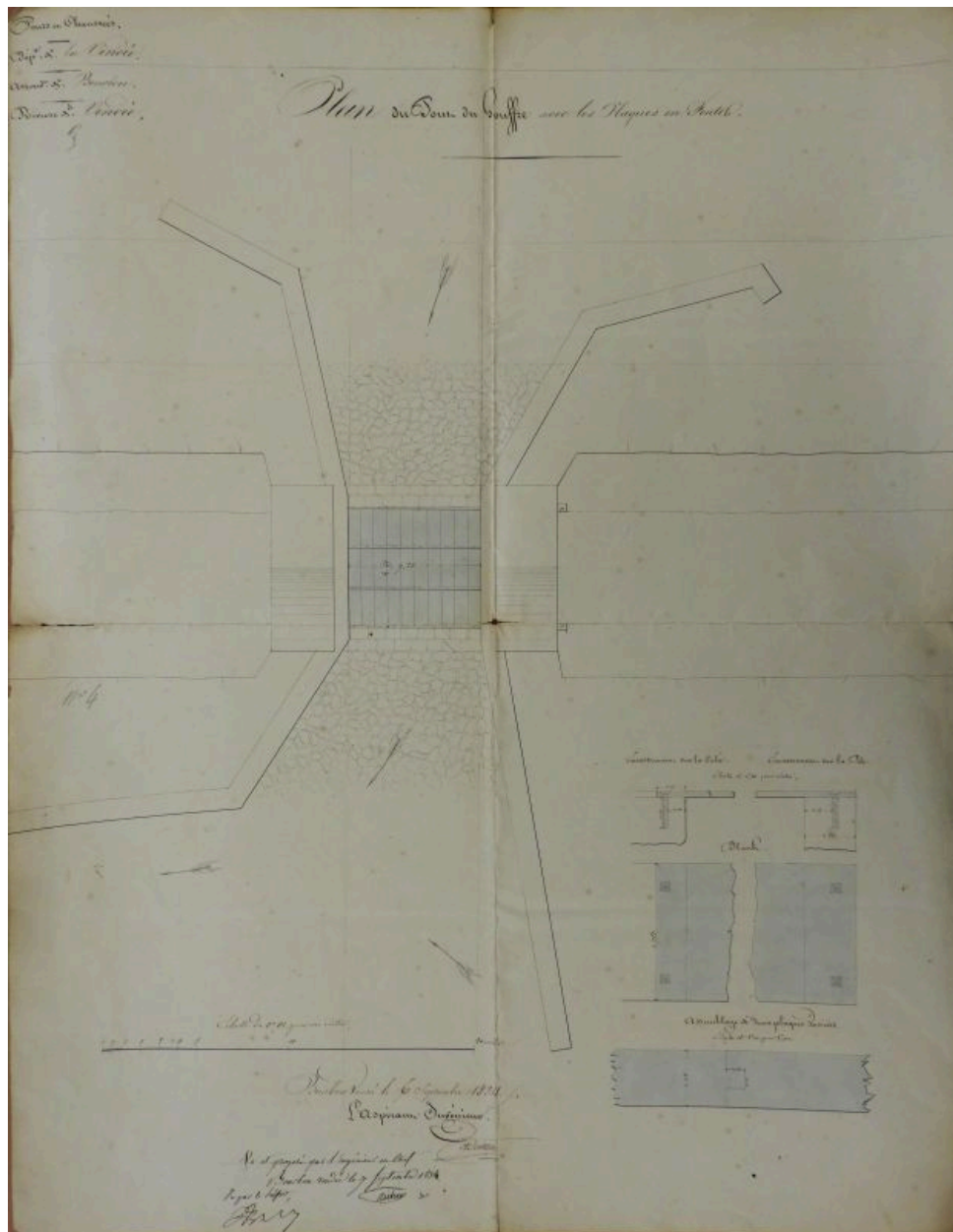
Plan de l'aqueduc du Gouffre avec radier en fonte, projet par Decharme, 6 septembre 1834.
