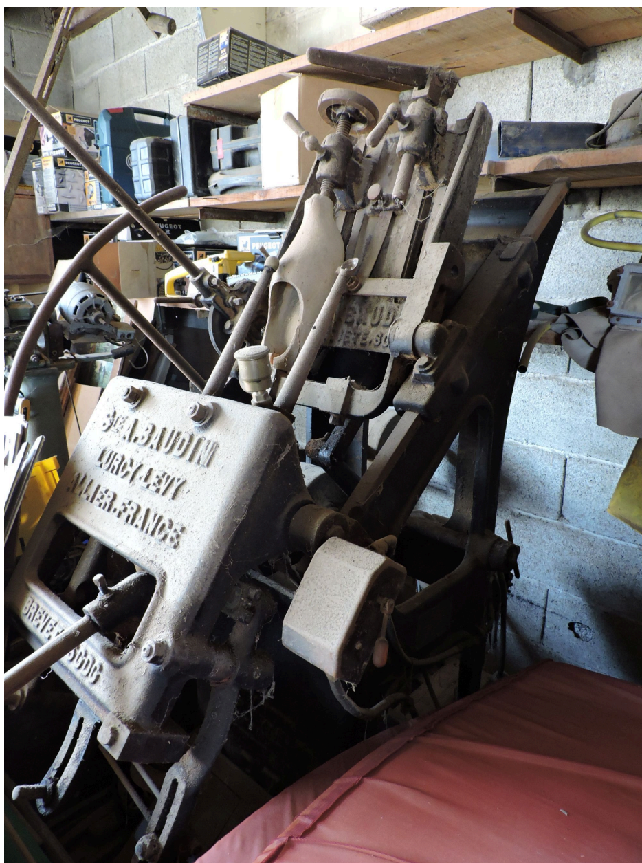
Détail de la machine.
