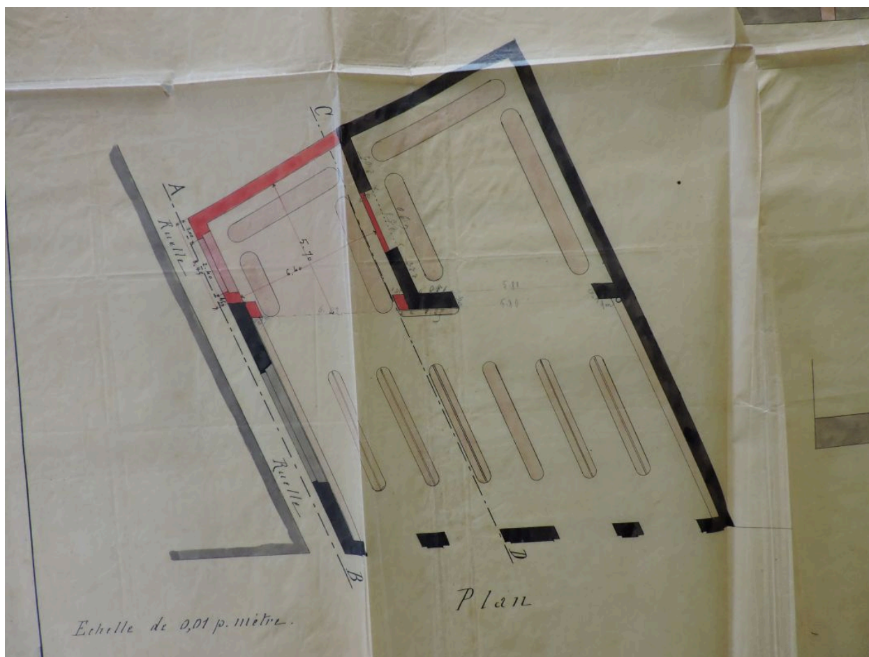
Projet d'agrandissement par Abel Filuzeau, 15 mai 1894 : plan.
