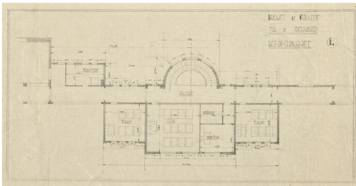
Projet de collège Notre-Dame de Béhuard. Rez-de-Chaussée. n.s. n.d.
