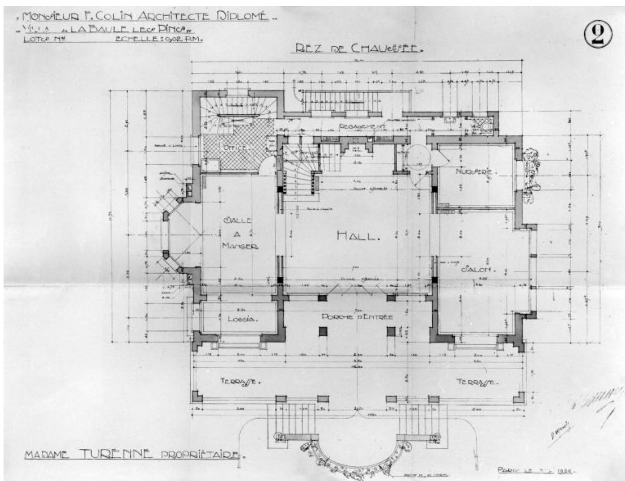
Plan du rez-de-chaussée au 1/50e de la villa Manégor dressée pour Madame Turenne.
