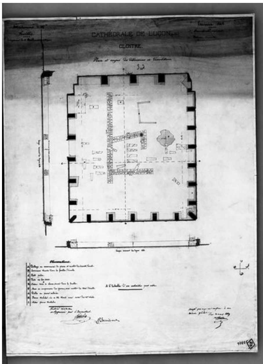
Plan et coupe des fouilles du cloître au 1/100e, par Emile Boeswillwald, en 1848.
