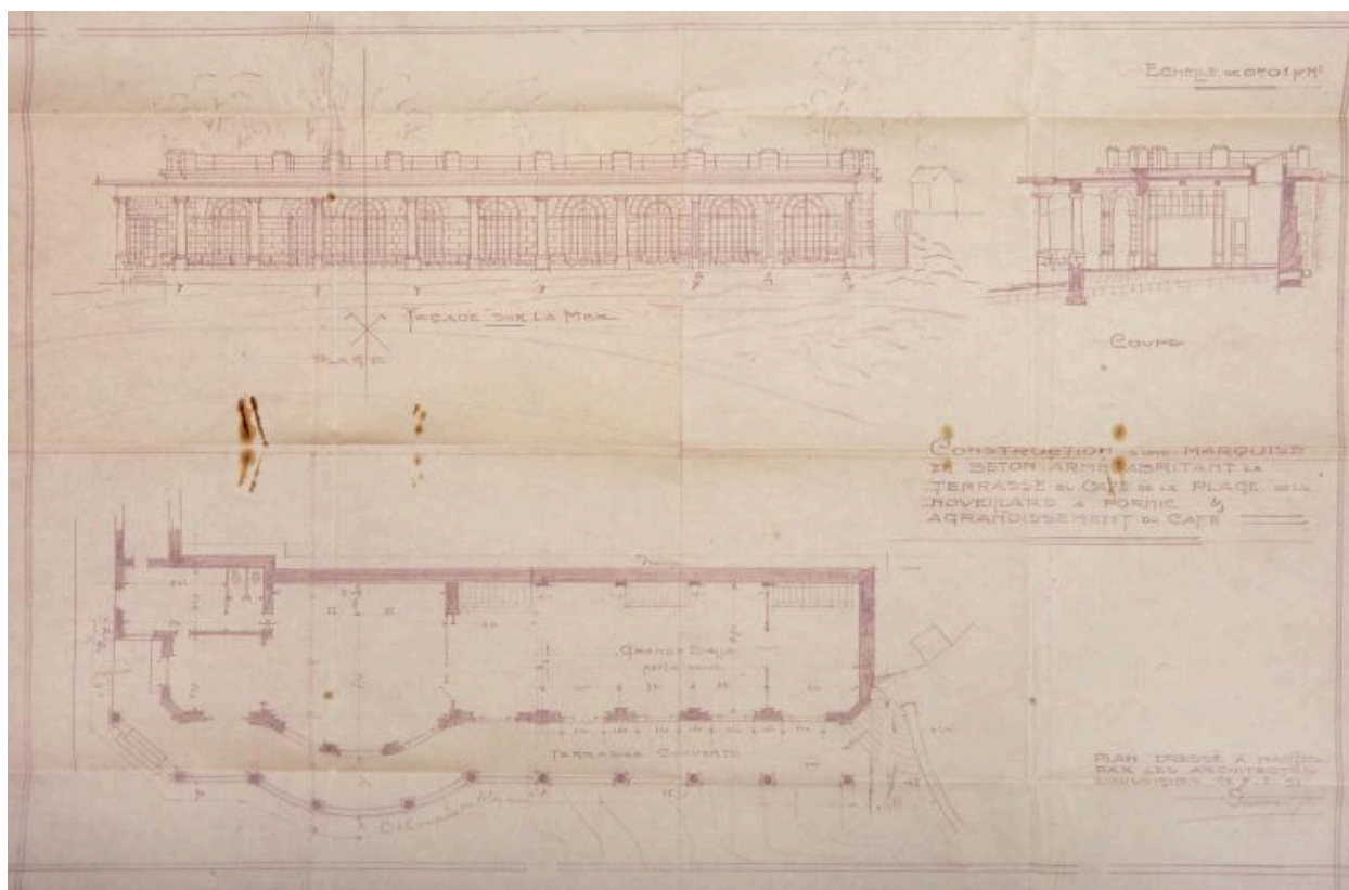
Plan et élévation, agrandissement du café, 1930.
