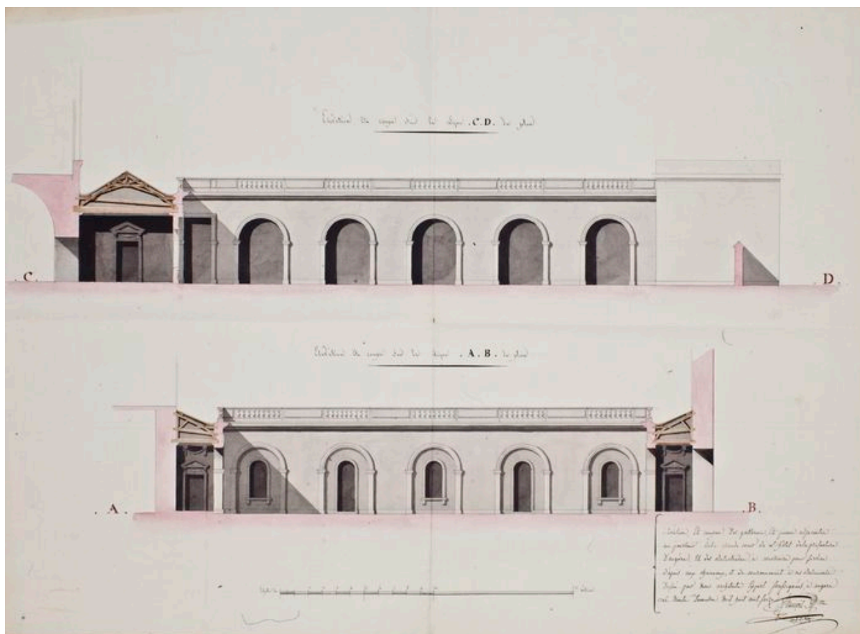
Galleries sur la cour d'honneur : projet de modification des couvertures et du couronnement (par des balustrades), élévations et coupes, par L. François, 1816. (Archives départementales de Maine-et-Loire ; N 1765).
