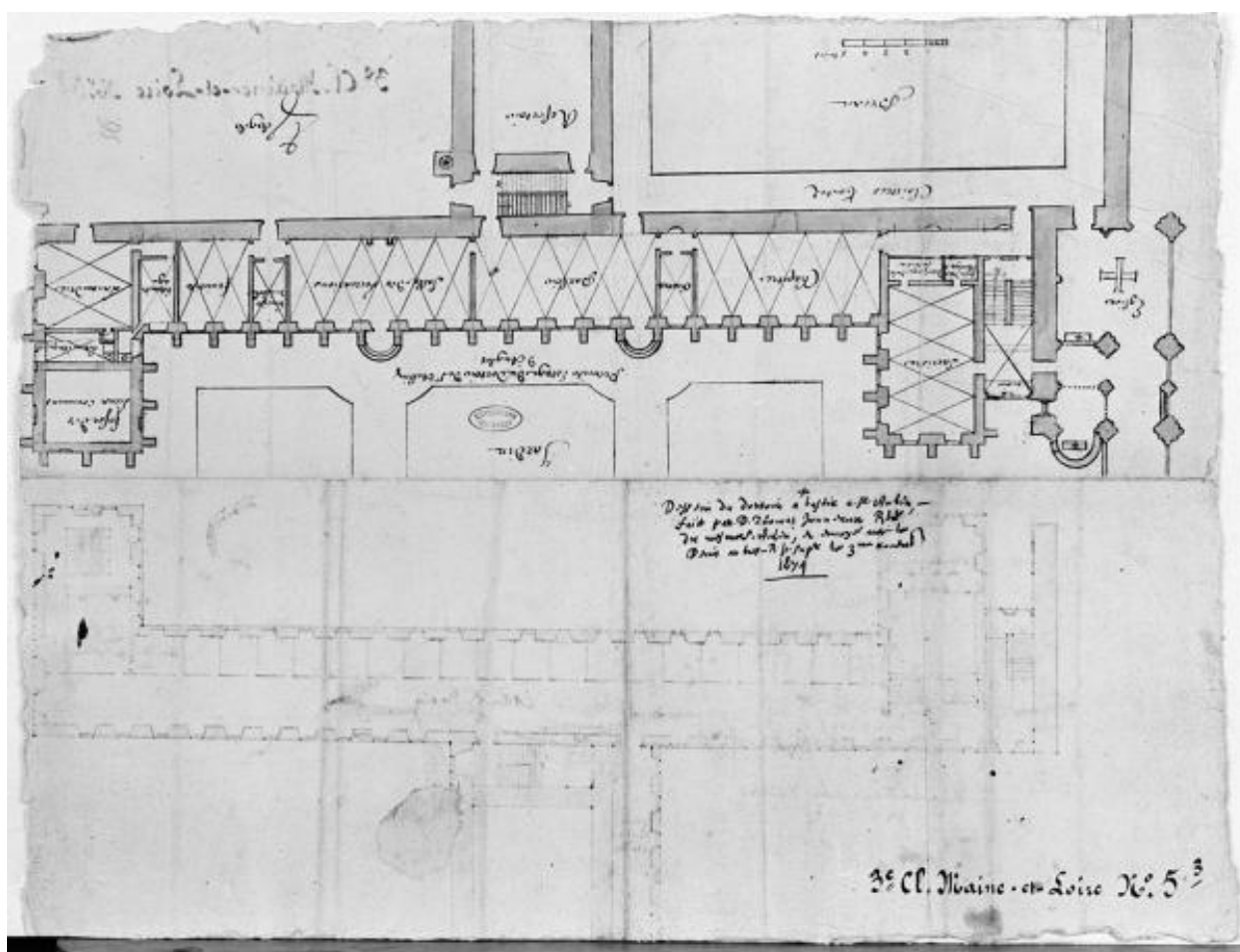
Dessin du dortoir à bâtir à Saint-Aubin, fait par Dom Journeaux...Premier étage... : plan au rez-de-chaussée de l'aile est. Lavis, 1674, éch. 1 : 243. (Archives nationales ; N III Maine-et-Loire 5/3, recto).
